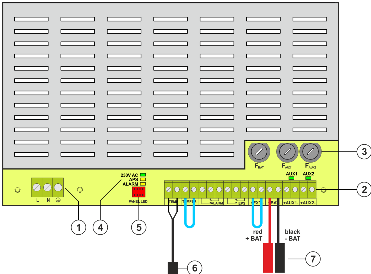
Obr. 2. Pohled na modul zdroje EN54C-2A7.
