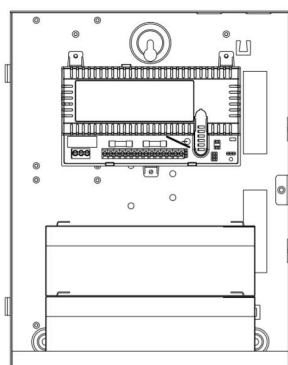
2401ST se skříní T a bateriemi 2,1Ah
