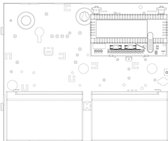
2401ST se skříní C a bateriemi 7Ah
