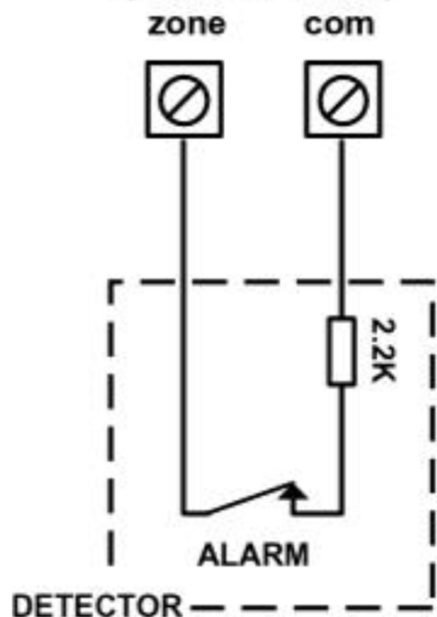
END OF LINE (EOL) RESISTOR (N.C. CONTACT)
